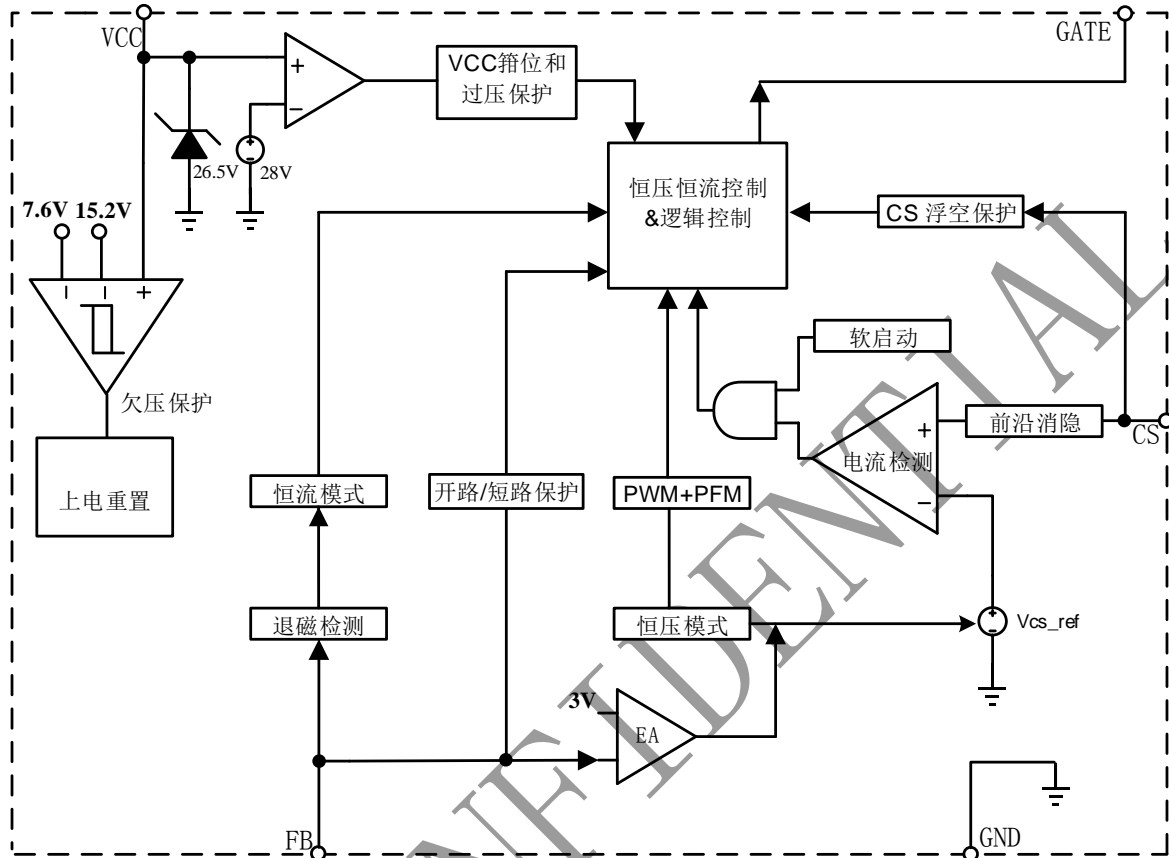
图 3 BP2519 内部框图
