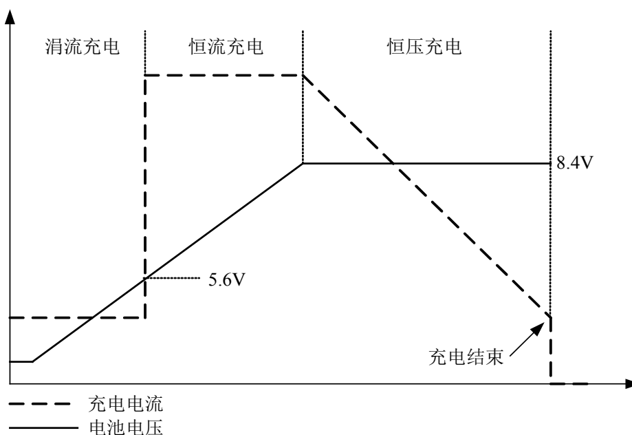
图2 充电过程示意图 (BAT 管脚直接连接到 FB 管脚)
